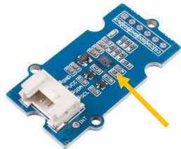
気圧・温度 センサ (DPS310)
